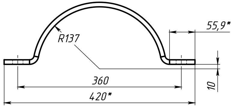
Поз.3 (Полухомут)
